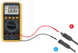
Figura 3.24 Medição com multímetro
